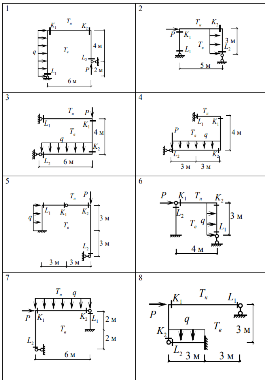
Рисунок 1 – Расчетная схема
