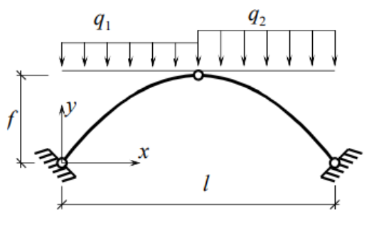
Рисунок 1 – Расчетная схема
