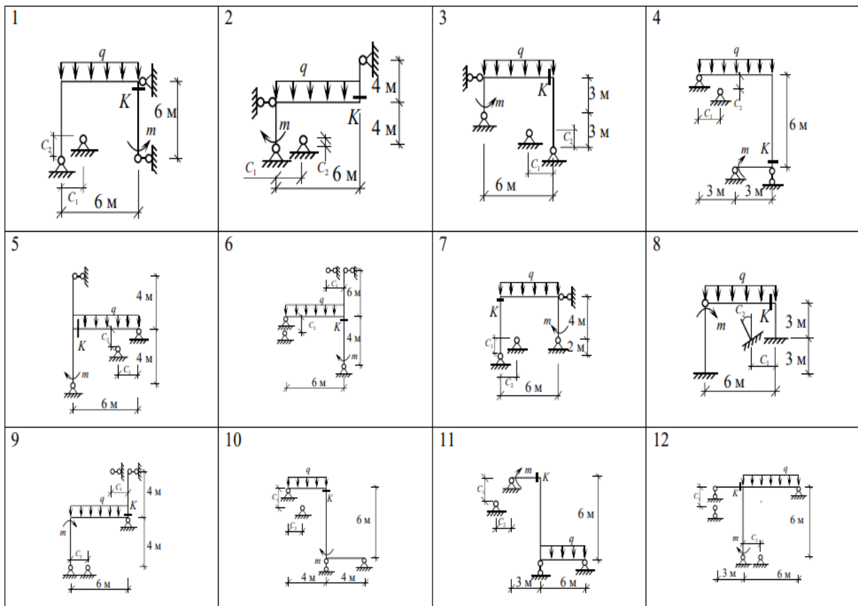
Рисунок 1 – Расчетная схема
