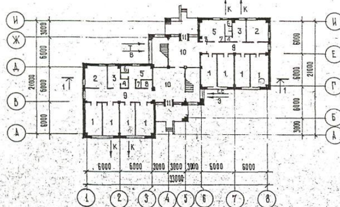
ПЛАН 2 ЭТАЖА
