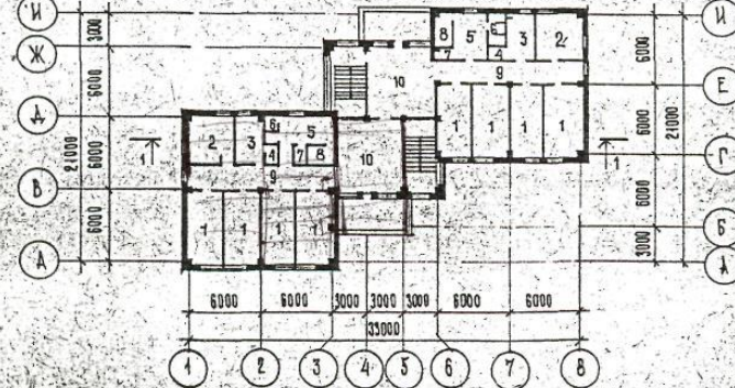
ПЛАН 2 ЭТАЖА
