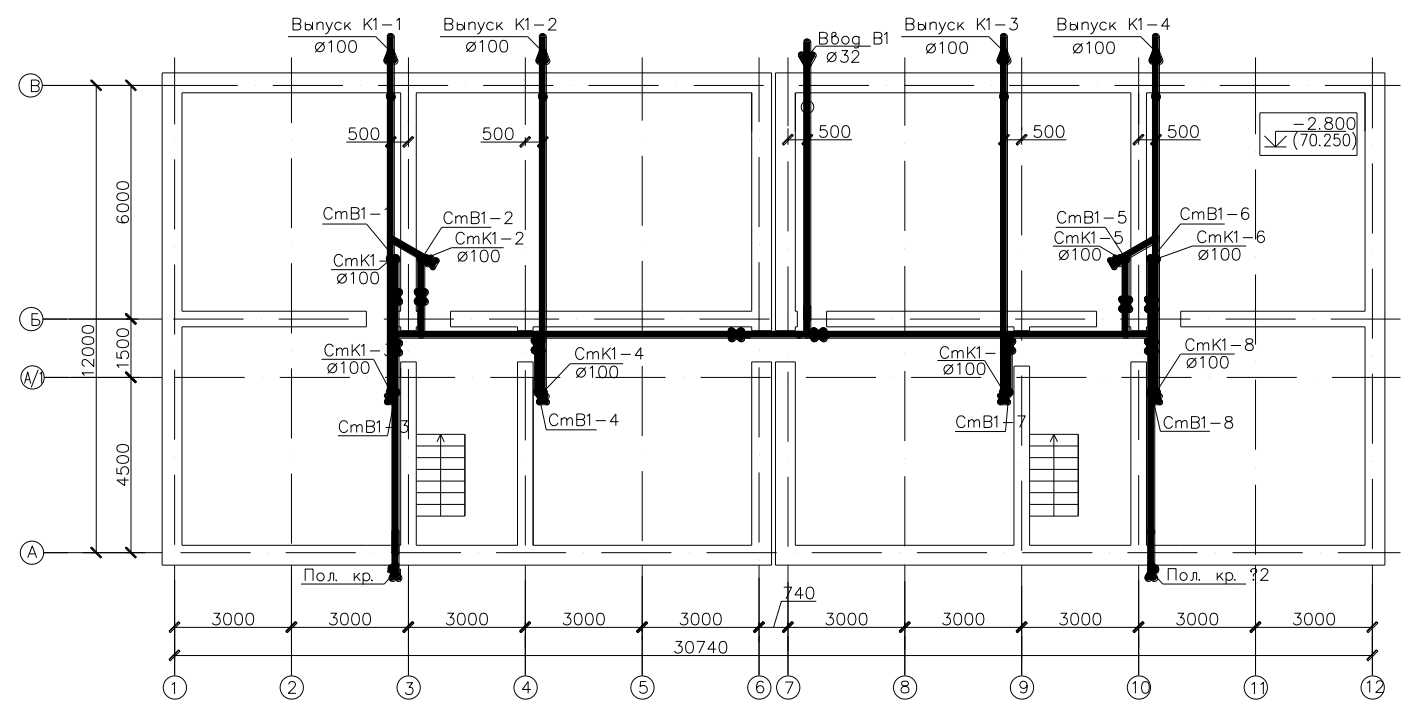
ПЛАН ПОДВАЛА
