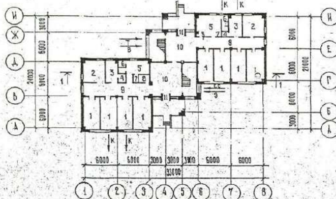
ПЛАН 2 ЭТАЖА
