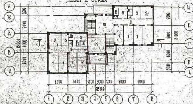
ПЛАН 2 ЭТАЖА
