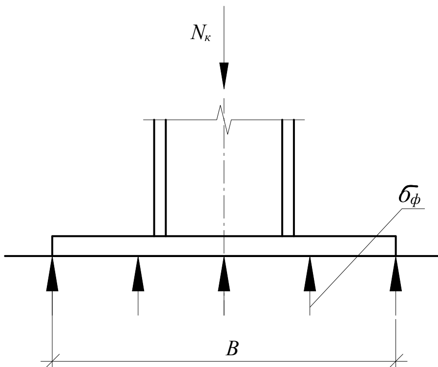
Рис. 16. К расчету опорной плиты
