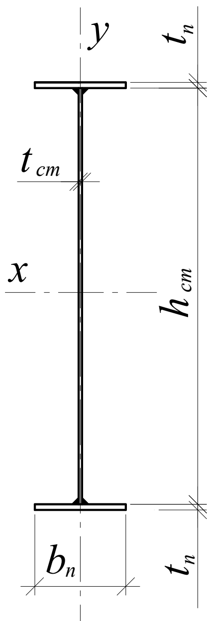
Рис. 3. Поперечное сечение главной балки
