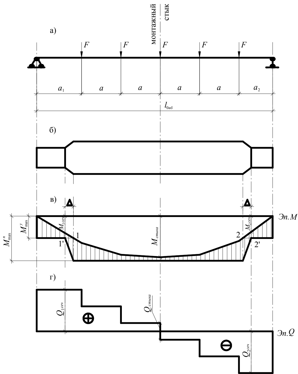
Рис. 5. Построение эпюры материалов: а) схема нагрузок; б) план балки; в) эпюры моментов и материалов; г) эпюра поперечных сил
