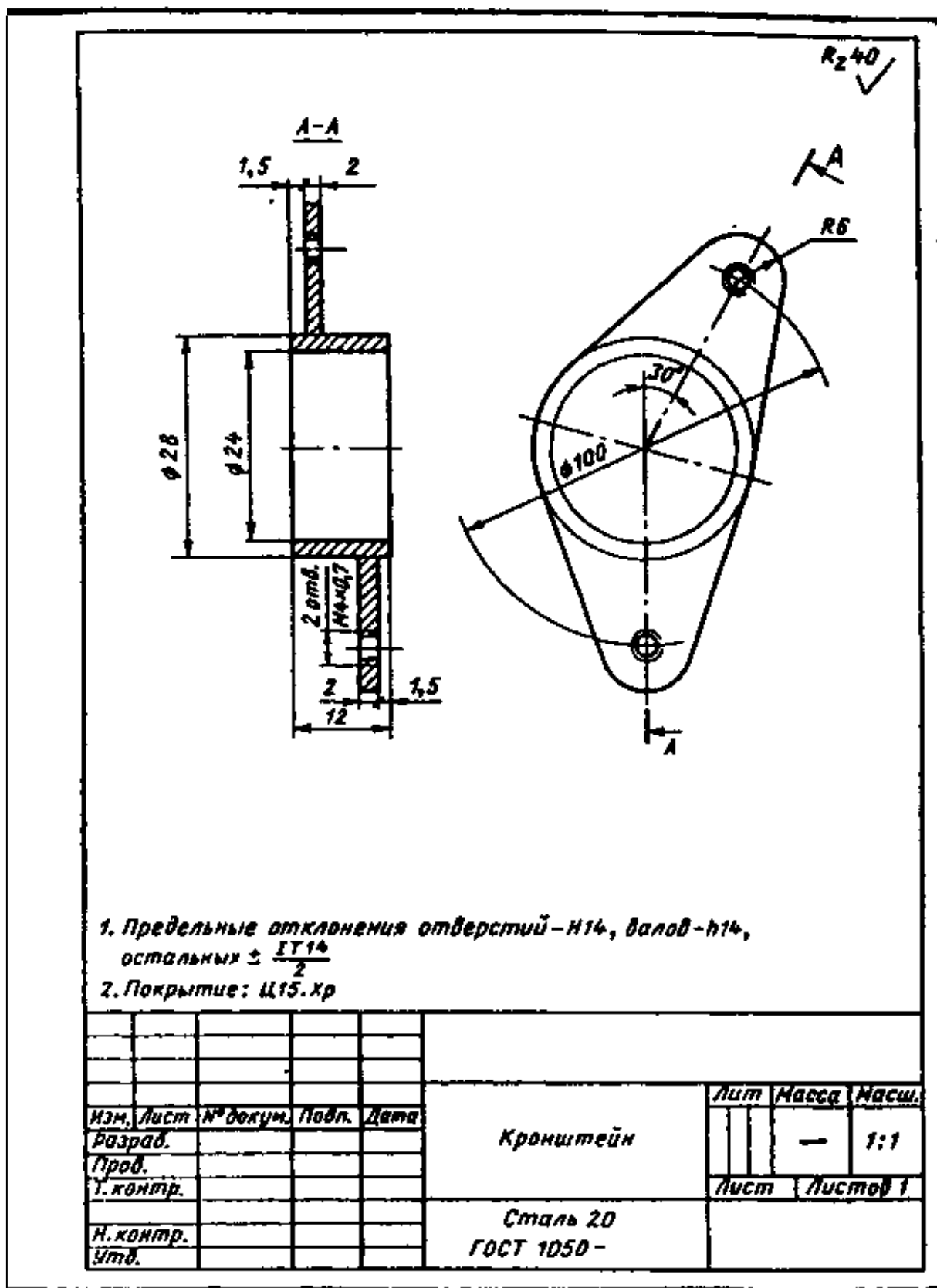
Рисунок 3- Пример оформления чертежа детали, формат А4
