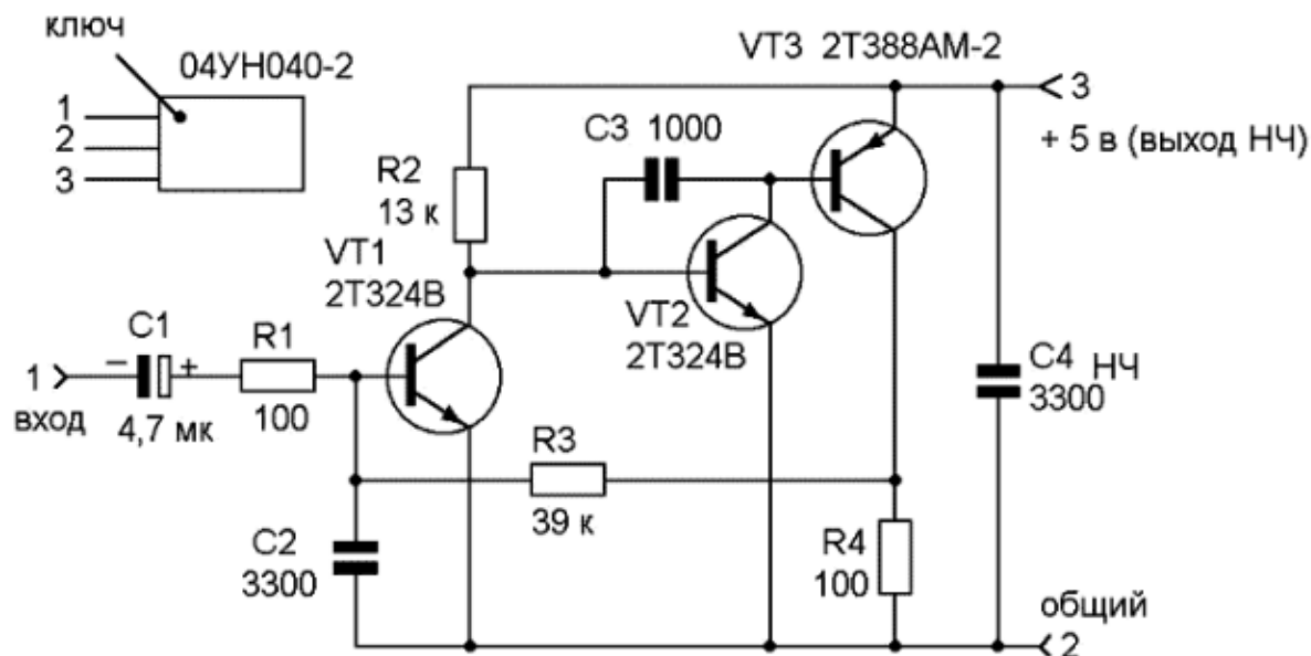
Схема пробника индикатора
