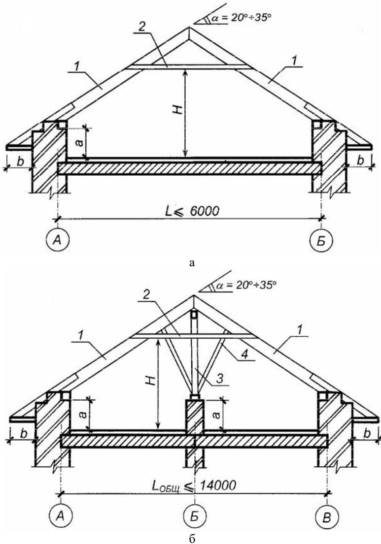
Рис.12.Конструктивные схемы скатных крыш: а–свисячим стропилами; б– наслонными стропилами;
