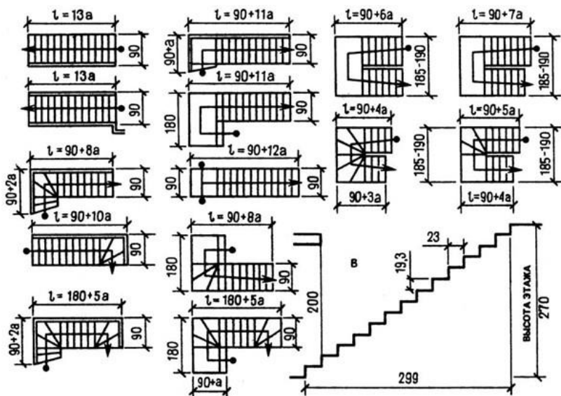
Рис. 5. Планировочные схемы различных типоввнутриквартирныхлестницс указаниемгабаритныхразмеров
