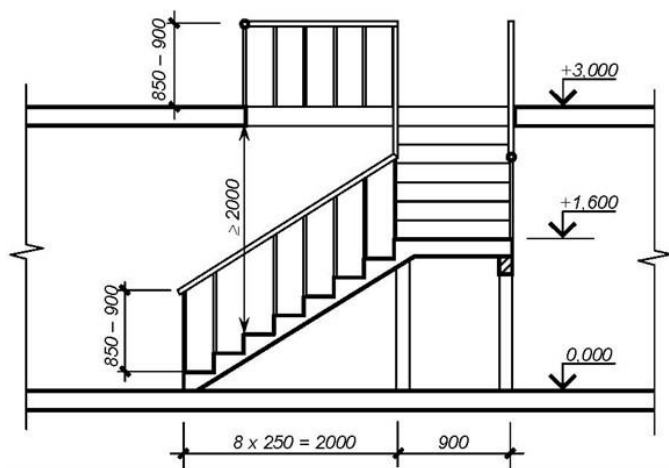
Рис.6.Схемавнутриквартирнойлестницисповоротомна90°: внижнеммарше8ступенейвысотой200мм,вверхнем–7 ступеней
