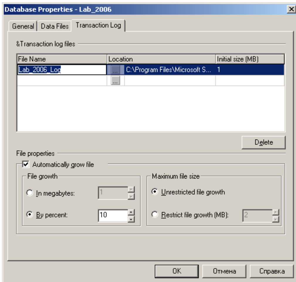
Рис 3.4. Вкладка Transaction_log
